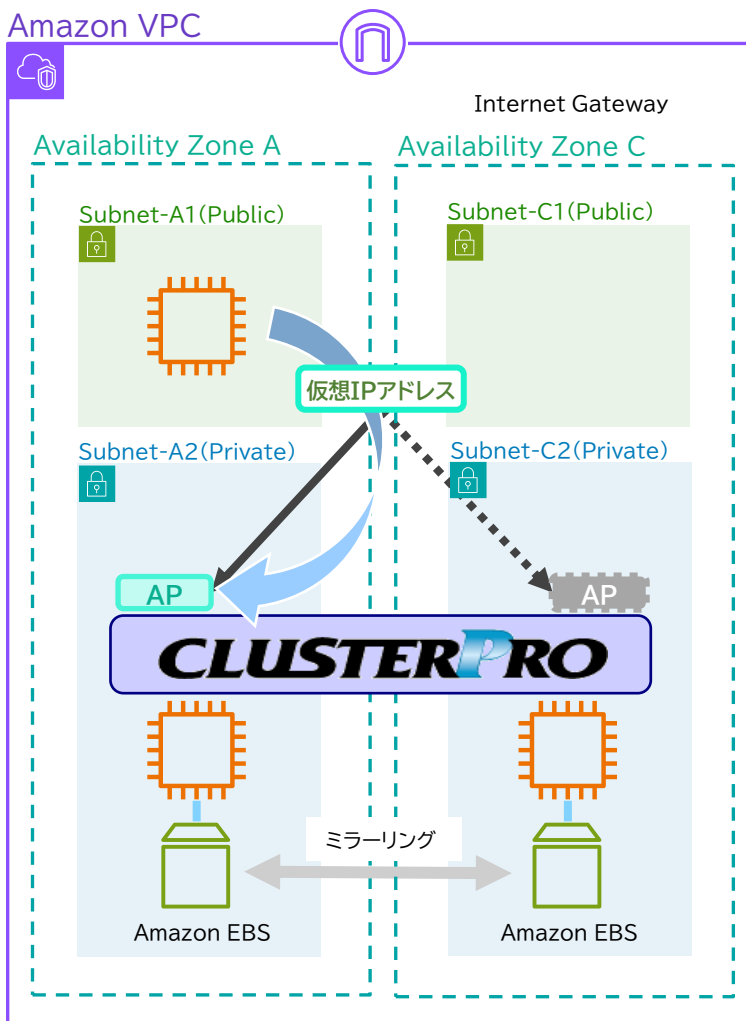
▼AWS環境でのCLUSTERPRO X 導入イメージ
