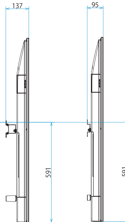
標準壁掛け (SU-WL450)
